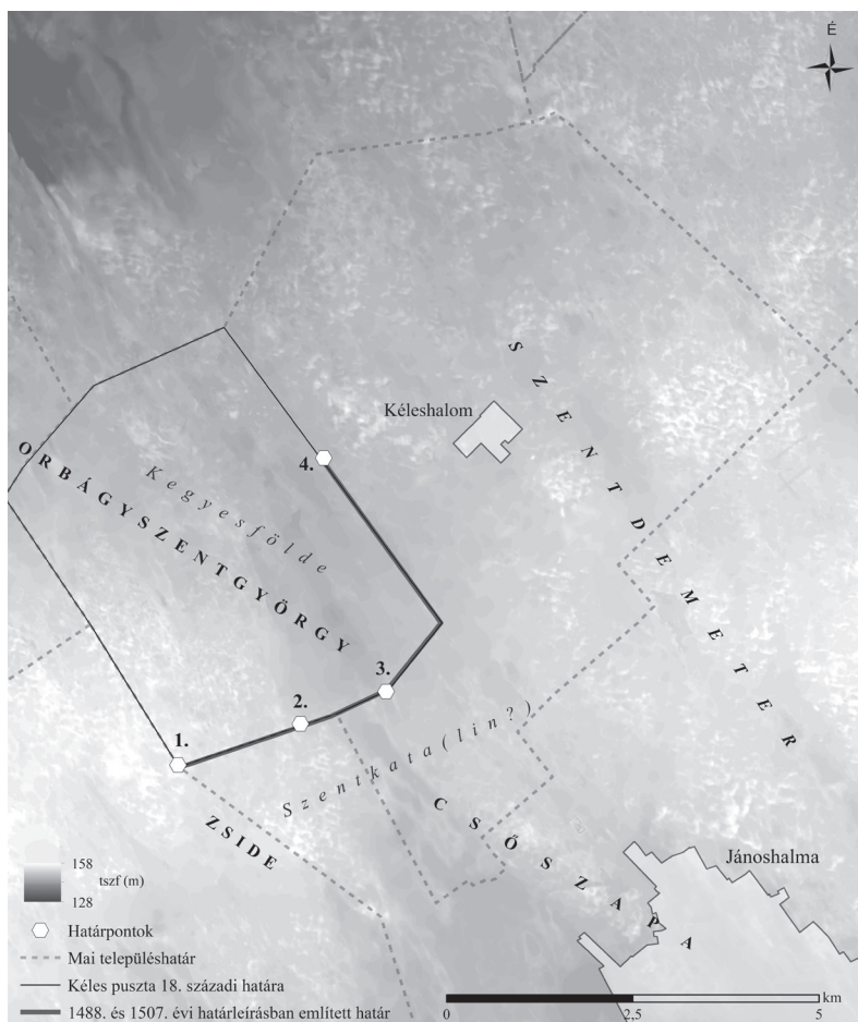
3. ábra: Kegyesfölde környezetének domborzati térképe (készítette: Pányi István) Figure 3 Topographic map of the surroundings of Kegyesfölde (Created by István Pányi)
