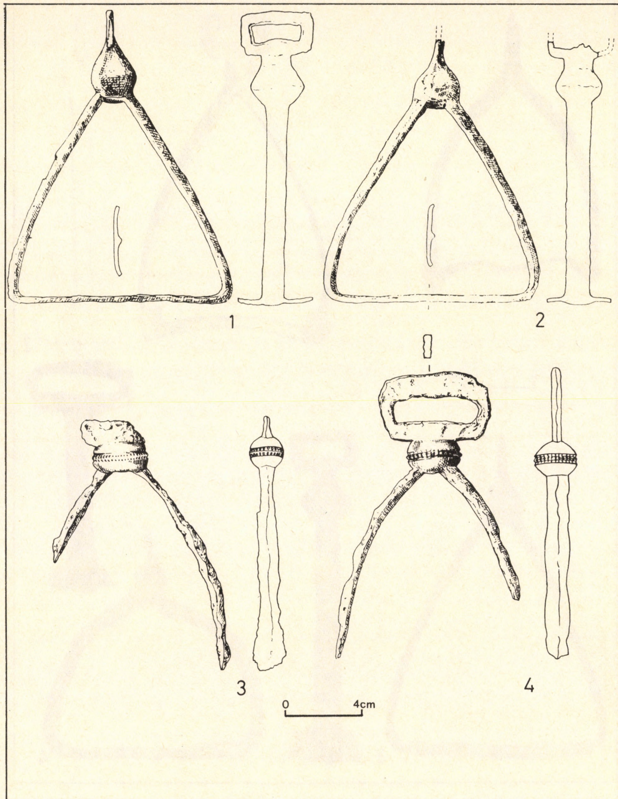
2. kép 1—4. A geszti gombos nyakú kengyelek (1—4.) Abb. 2. 1—4. Die Steigbügel von Geszt mit knopfförmigem Hals (1—4.)
