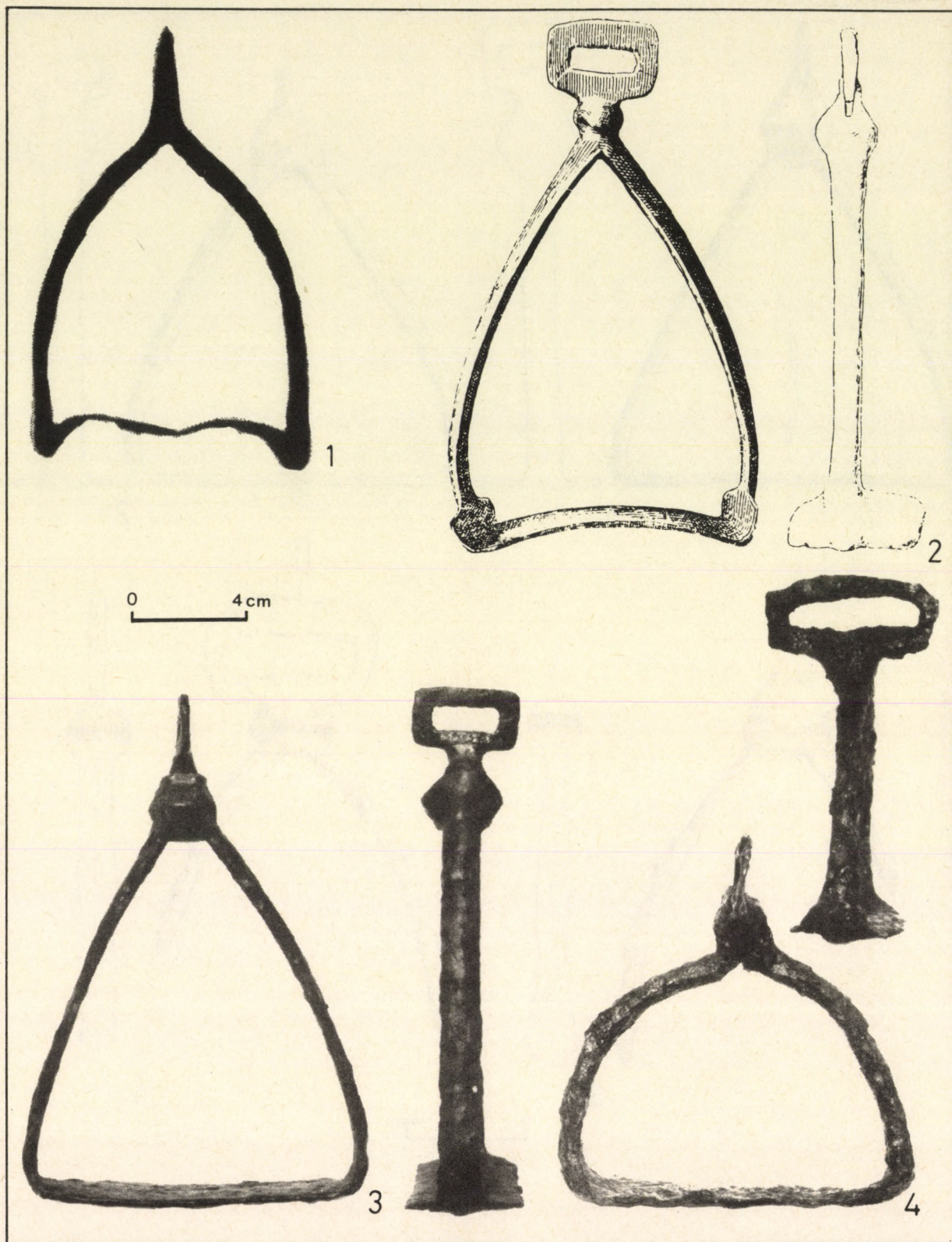
3. kép 1—3. Ismeretlen lelőhelyű (5—7.) és 4. a koroncó—rácdombi (8.) gombos nyakú kengyel Abb. 3. 1—3. Von unbekanntem Fundort (5—7.) und 4. der Steigbügel von Koroncó—Rácdomb (8.) mit knopfförmigem Hals
