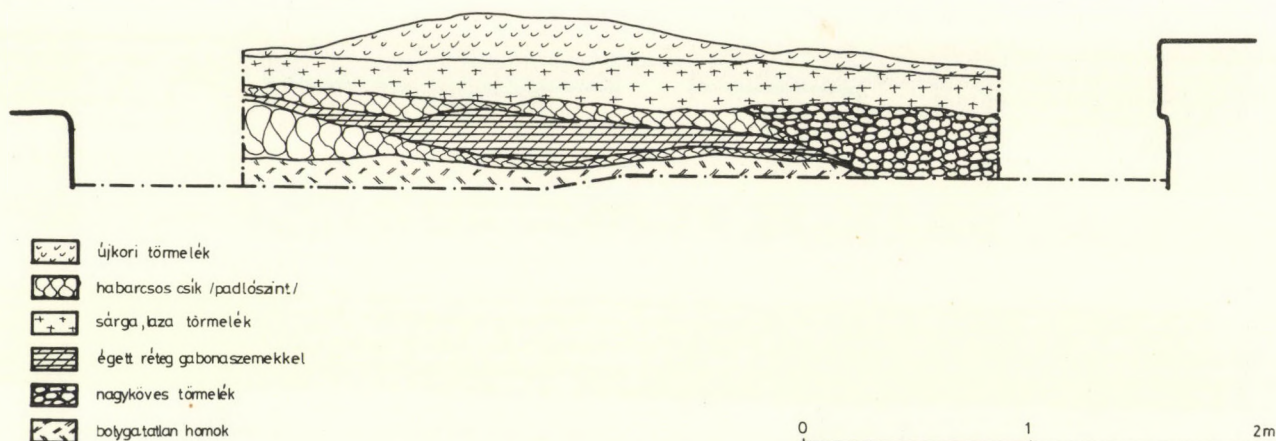
33. kép I—I metszet az égett gabonarétegről
