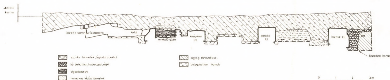
20. kép C—C metszet, a 15. kutatóárok keleti faláról.
