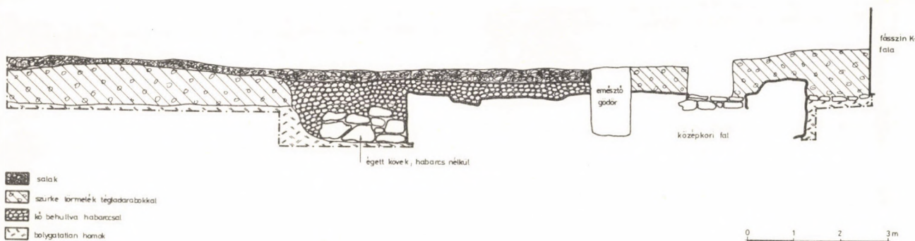
28. kép F–F metszet a 14. kutatóárok déli faláról.
