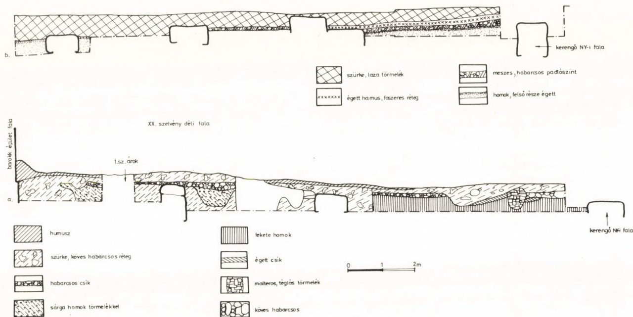
31. kép a) G—G metszet a monostorudvarról; b) H—H metszet a monostor nyugati szárnyáról.
