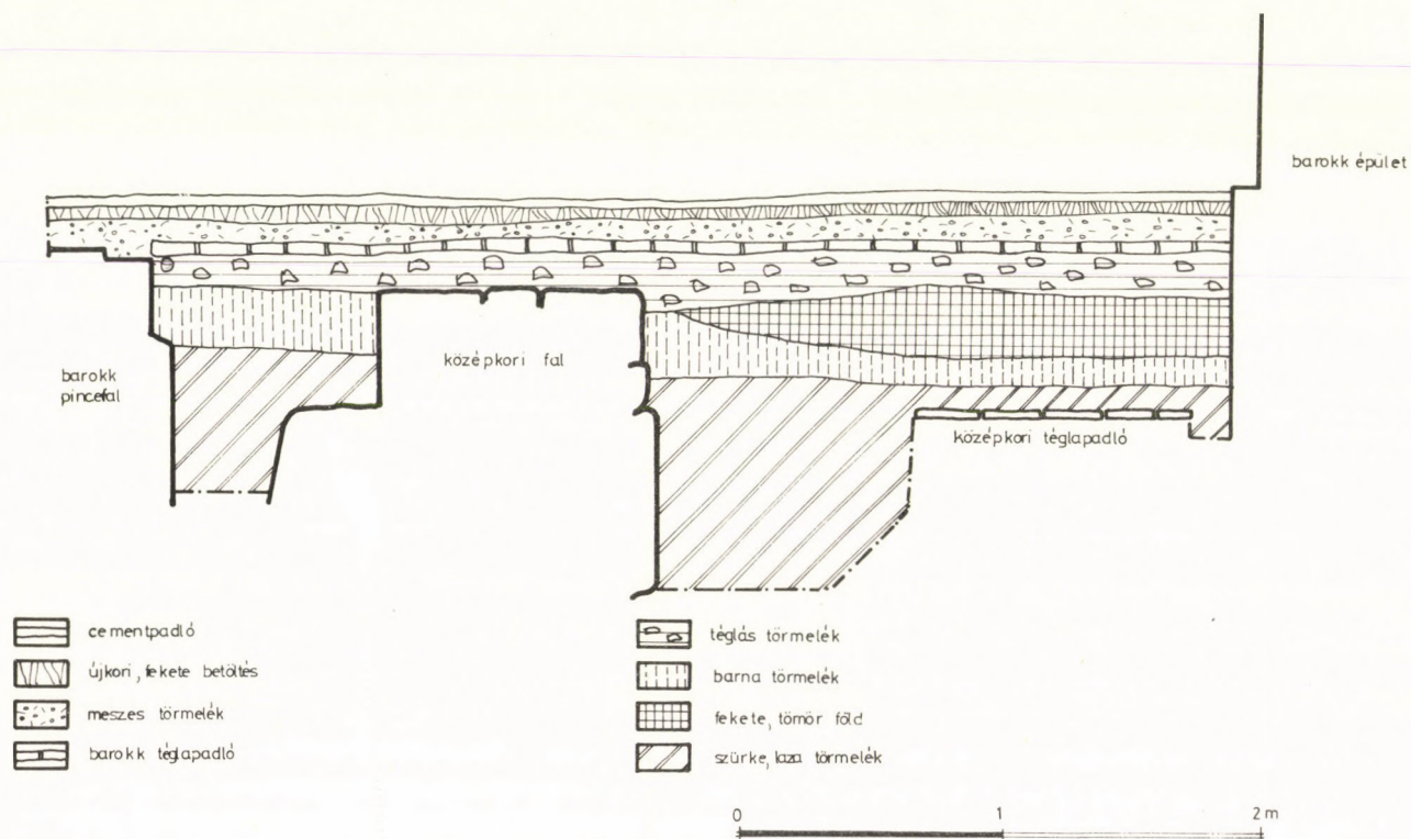
22. kép D—D metszet a 8. kutatóárok nyugati faláról.
