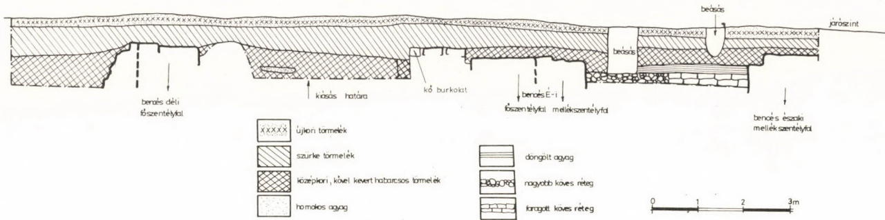
8. kép A—A metszet.
