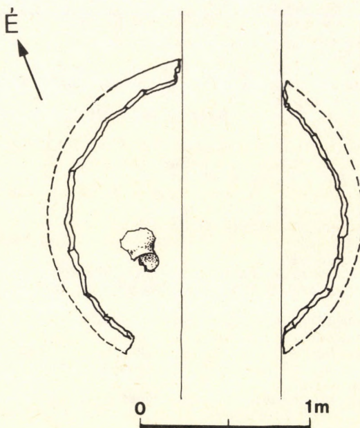
2. kép Esztergom-Diósvölgy. A kemence alap- és metszetrajza (1 : 25) Abb. 2. Esztergom-Diósvölgy. Grundriß- und Profilzeichnungen des Ofens (1:25)
