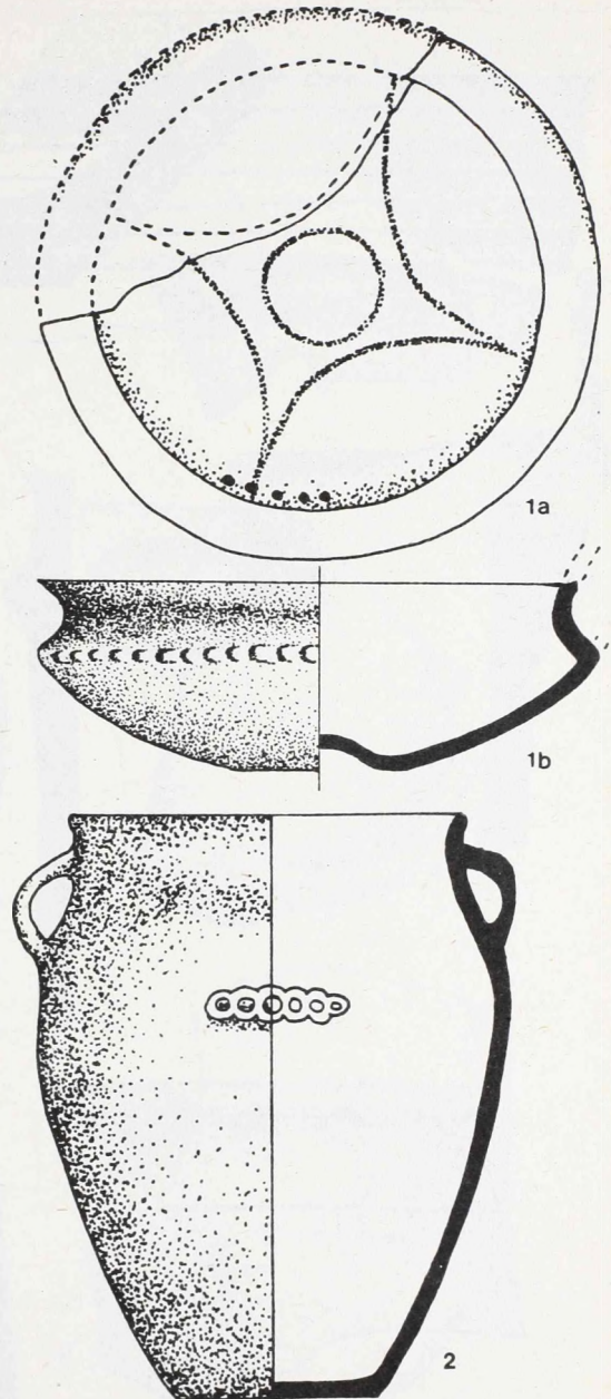
11. kép 1: díszített korsóska a depotból; 2: fazék a depotból Abb. 11. 1: Verzierter Krüggchen aus dem Depot, 2: Topf aus der Grube H = 1 = 1:2; 2 = 1:3
