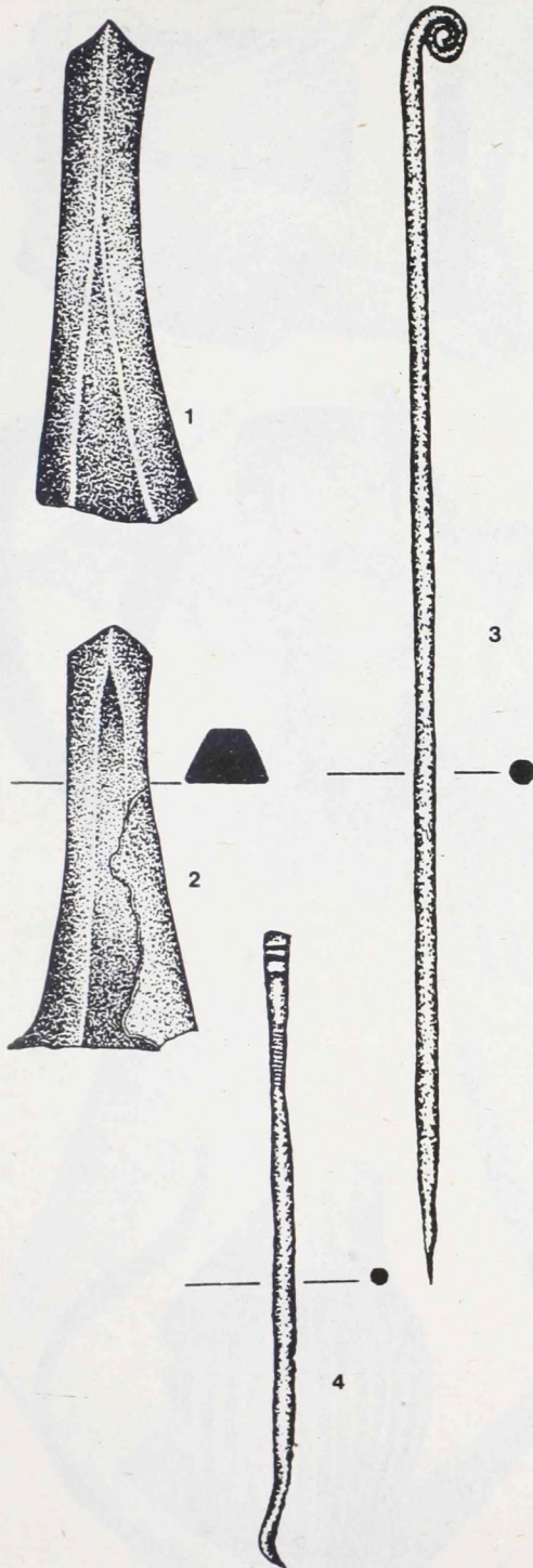
10. kép Fültörédekek és tűk a gödörből Abb. 10. Henkelfragmente und Nadeln aus der Grube H = 1-4 = 1:1
