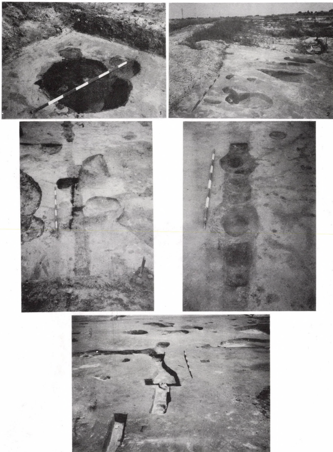
6. kép 1: az Északi szelvény szabadtéri tüzelőhelyei feltárás közben; 2: a 48. tüzelőgödör feltárás közben; 3: a 4. ház északi falának alapozási árka; 4: az egyik cölöplyukba törött gerenda a 4. ház északi alapozási árkában; 5: a 4. ház DK-i sarka, az alapozási árok feltárás után
