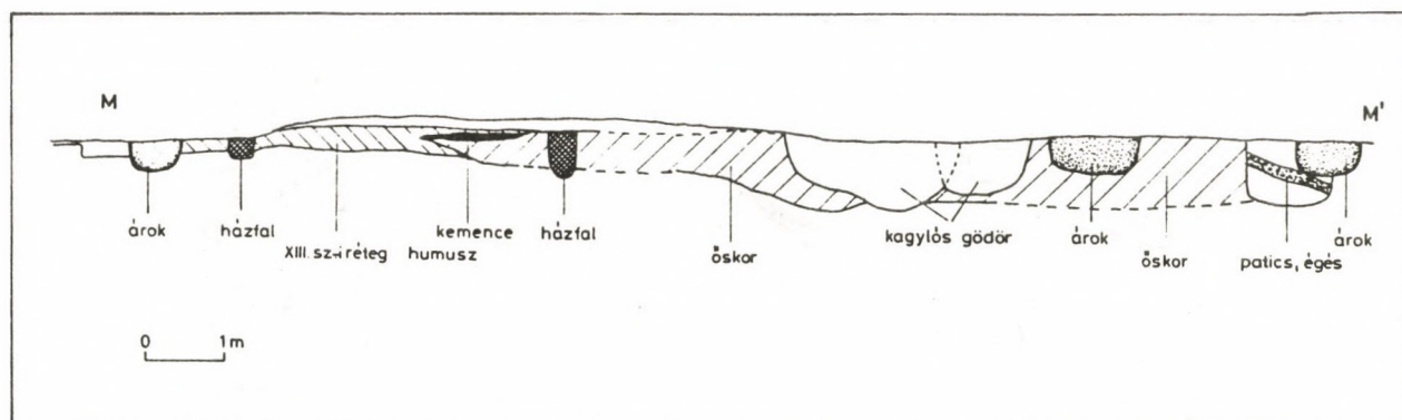
4. kép Az I. szelvény Ny-i felének metszetrajza Figure 4. Le dessin de section du mur ouest du segment 1.
