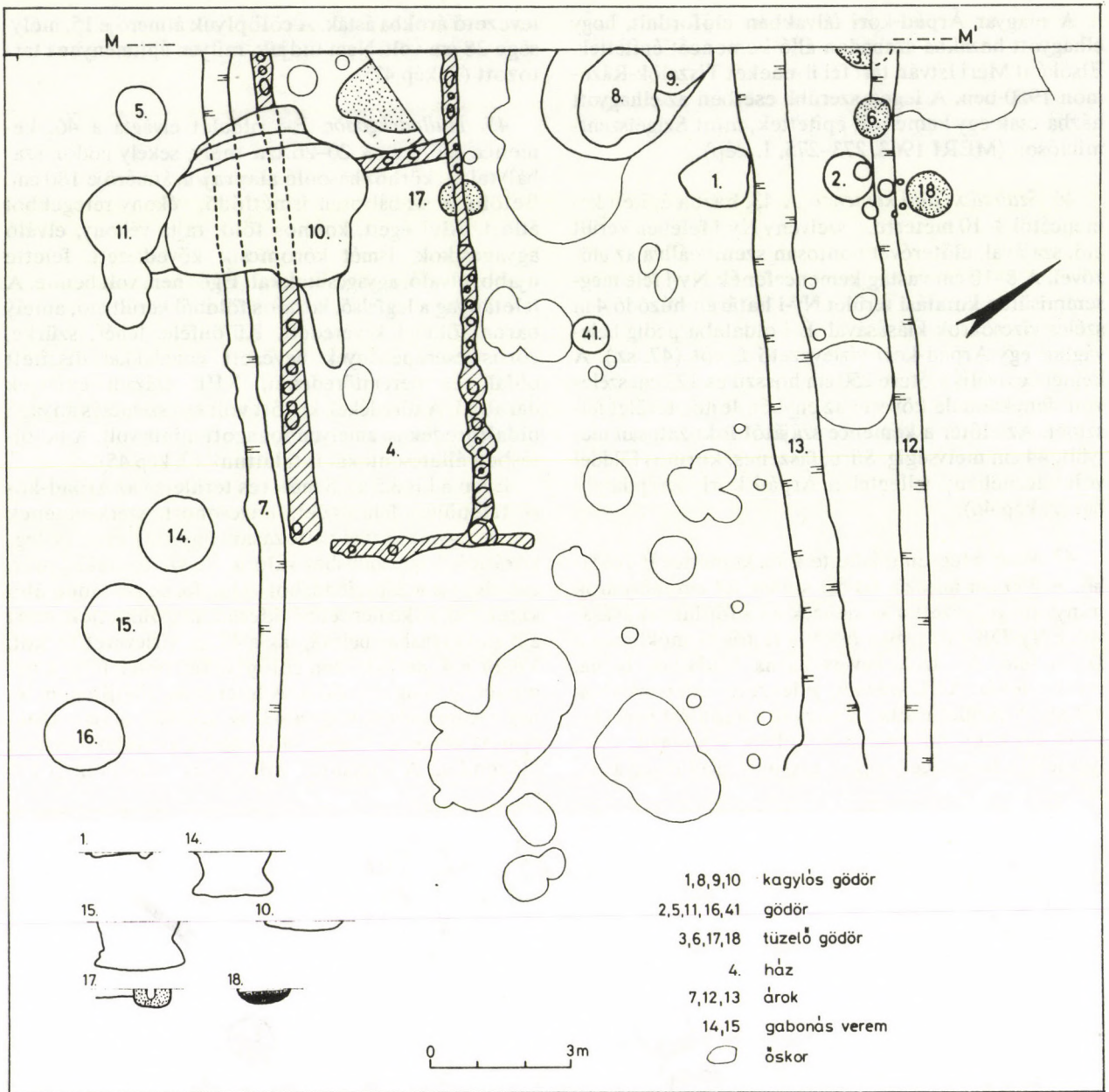
3. kép Az I. szelvény déli felében feltárt XIII. századi lakóház, és a körülötte lévő építmények helyszínrajza Figure 3. Le plan de la maison du 13 e siècle découverte à côté sud du segment avec les établissements qui l'entourent
